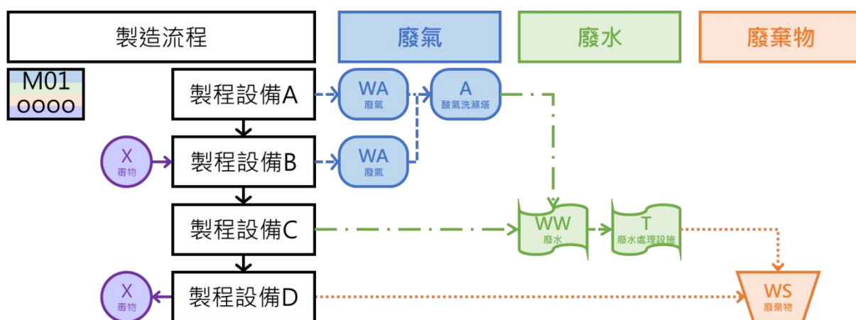
圖一、空、水、廢、毒化物污染流向圖（示意圖）
